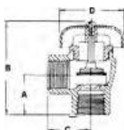
AVB1 38/38LF-10X
