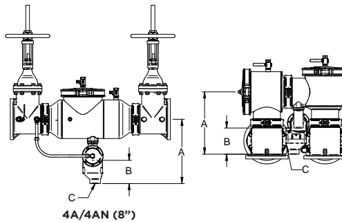
4A/4AN (8")
