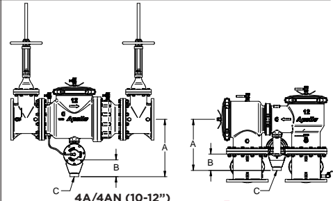
4A/4AN (10-12")
