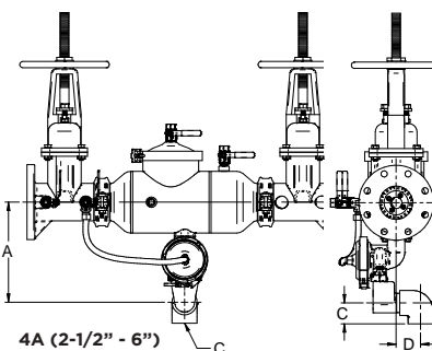
4A (2-1/2" - 6")
