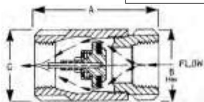
61-500
